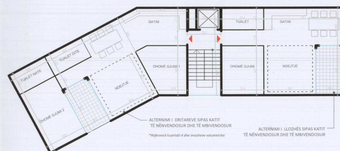
PLANIMETRI SKEMATIKE TE KATEVE TIP_GODINA D
