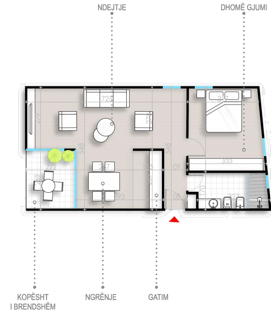
AP TIP [13] 1+1 SIPËRFAQE BRUTO: 69.6 m 2 SIPËRFAQE NETO: 60 m 2
