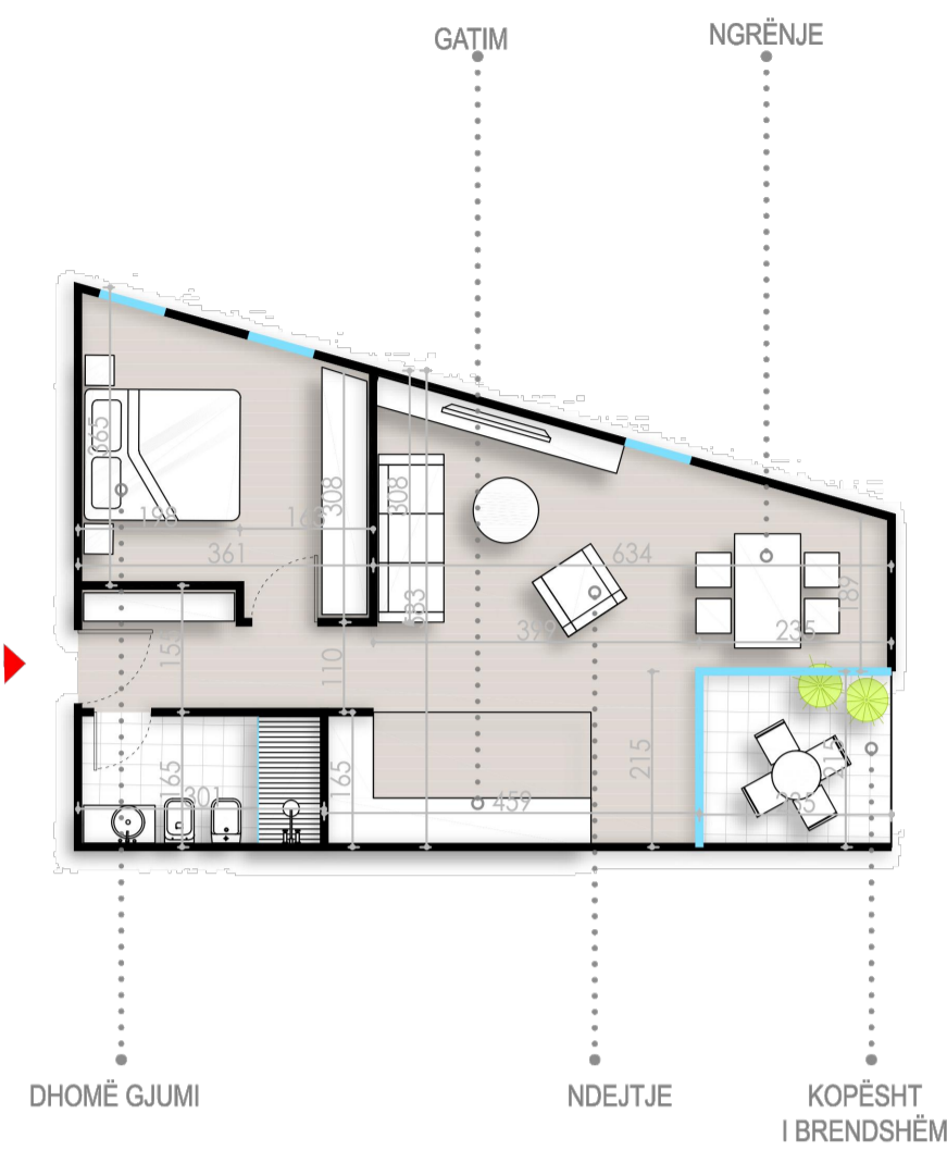
AP TIP [11] 1+1 SIPËRFAQE BRUTO: 63.8 m 2 SIPËRFAQE NETO: 55 m 2
