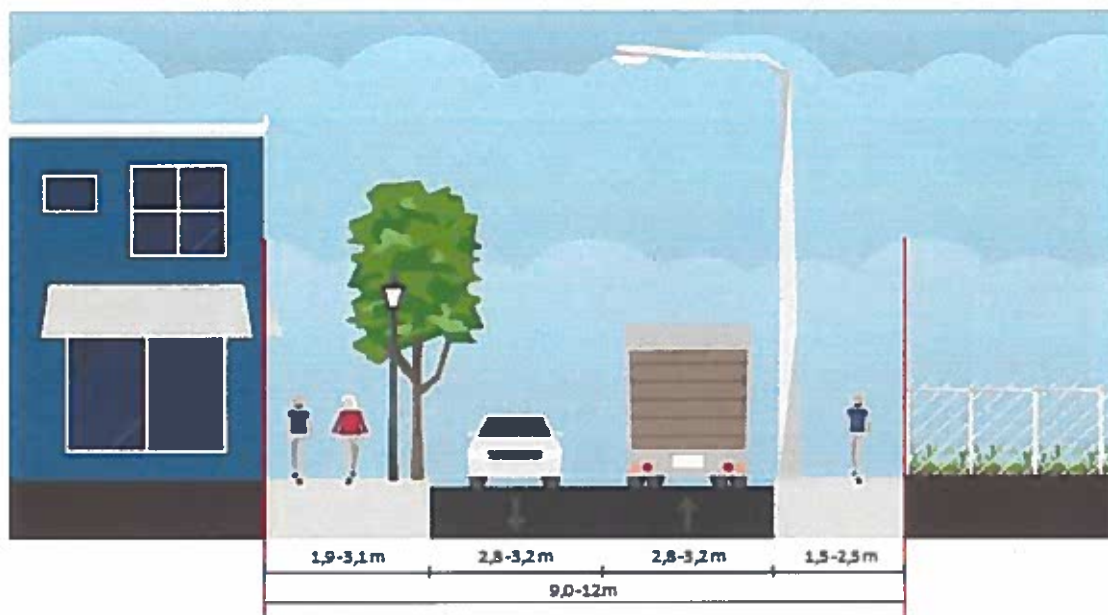
RRUGË URBANE DYTËSORE (E), 9-12m
