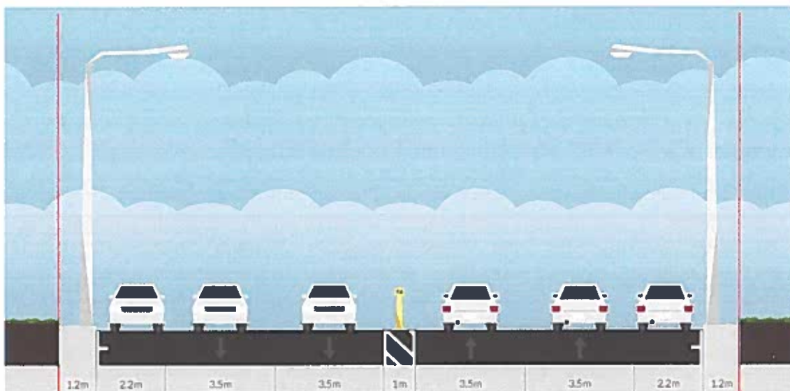
Figure 1. Rrugë interurbane kryesore e kategorisë B
