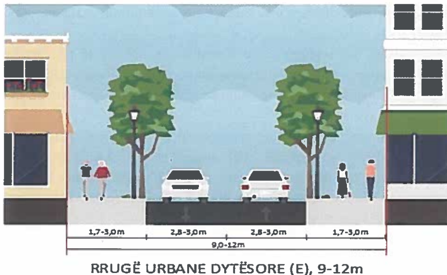
Figure 3. Rrugë urbane dytësore e kategorisë E (I)
